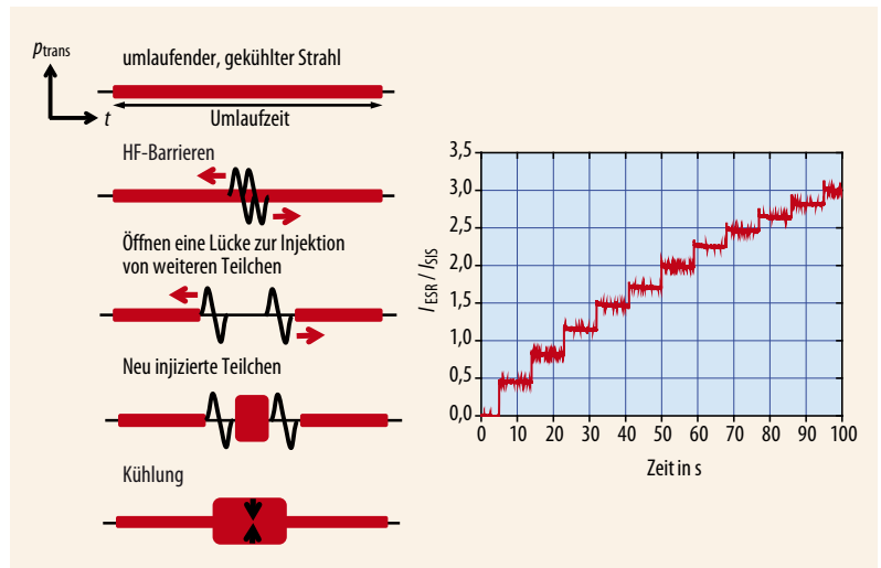
Abb. 4 Einfangs- und Kühlszenario zur Akkumulation von Teilchen in den Speicherringen HESR und NESR (links) und Messungen zum Test der Methode im ESR der GSI (rechts). Die Teilchen vertei-
