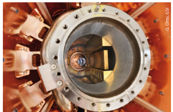
Abb. 3 Der Kryo-Kollimator für den geplanten supraleitenden FAIR-Beschleuniger SIS100 besitzt eine Goldbeschichtung, die dafür sorgt, dass beim Auftreffen von Strahlteilchen möglichst wenige Teilchen ins Strahlrohr abgegeben werden. Das ermöglicht ein stabiles Vakuum im Beschleuniger und hohe Strahlintensitäten im Schwerionenbetrieb.
