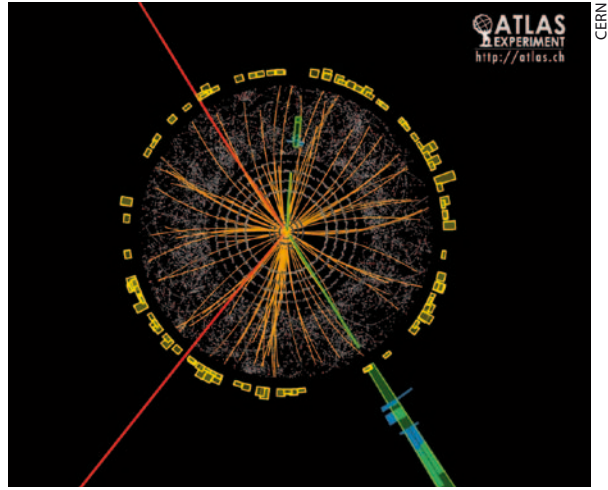
Der Zerfall eines Higgs-Boson-Kandidaten in zwei Photonen (links, CMS) oder vier Leptonen (rechts, ATLAS) lässt sich besonders eindeutig nachweisen.
